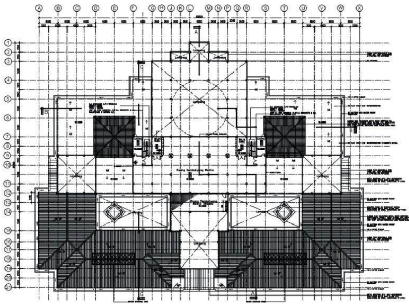
PELAN LANTAI ARAS MEZANIN (RUANG SEMBAHYANG WANITA)
